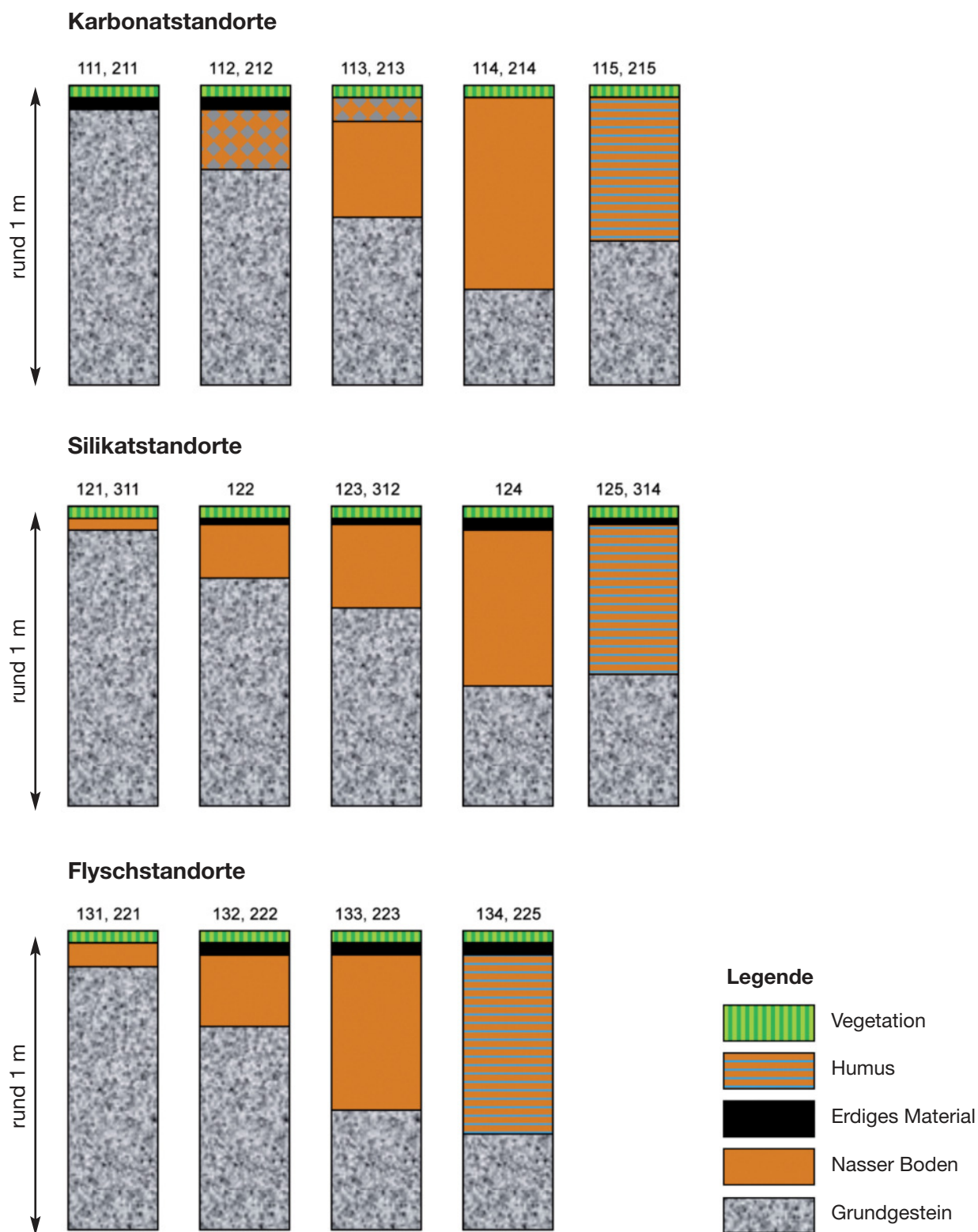
Abbildung 6: Schematische Bodenprofile
