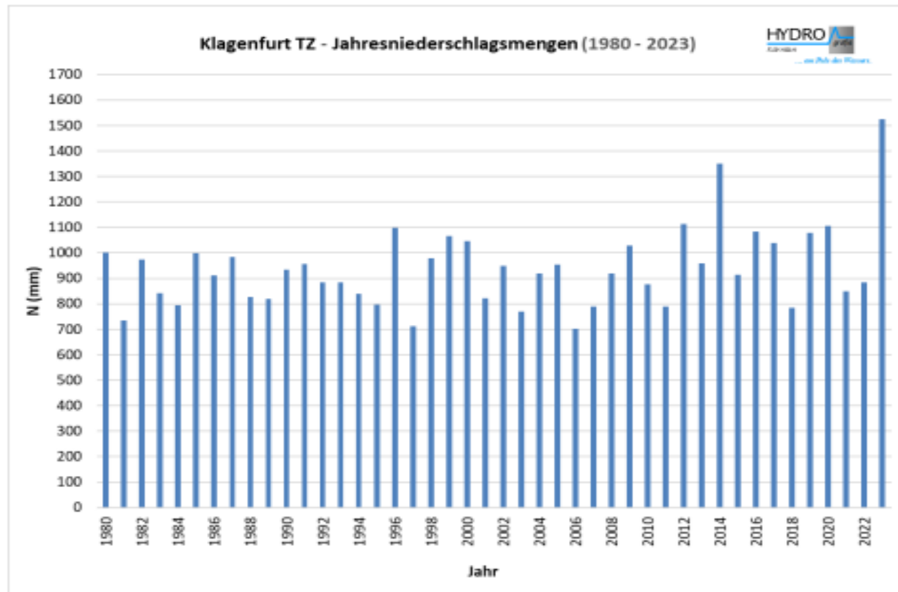
Abb. 12: Jahresniederschlagssummen in Klagenfurt 1980 – 2023; Hydrographischer Dienst Kärnten
